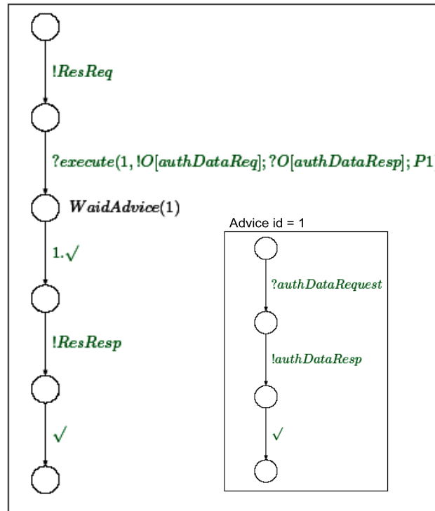
Figure 5. L'automate du client dynamique.
