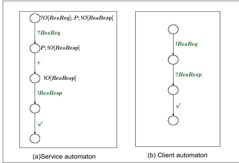
Figure 2. Les automates service et client du processus des analyses sanguines.
