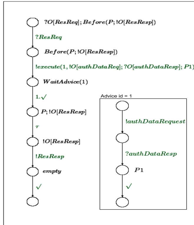
Figure 4. L'automate du processus adaptable.
