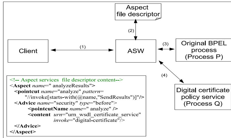
Figure 1. Le schéma d'interaction pour l'insertion d'une politique de sécurité.
