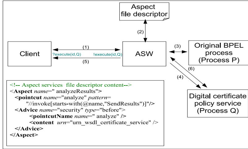
Figure 3. Le nouveau schéma d'interaction pour l'insertion d'une politique de sécurité.
